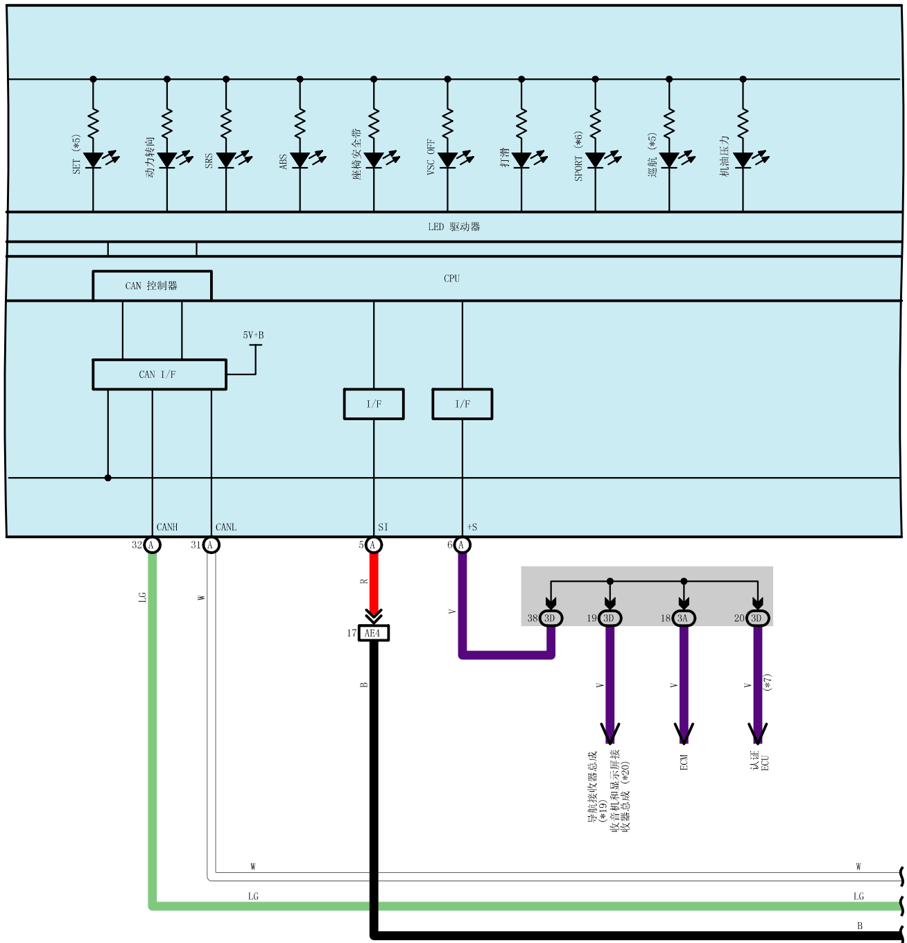
E55 (A), E59 (B) 组合仪表总成
