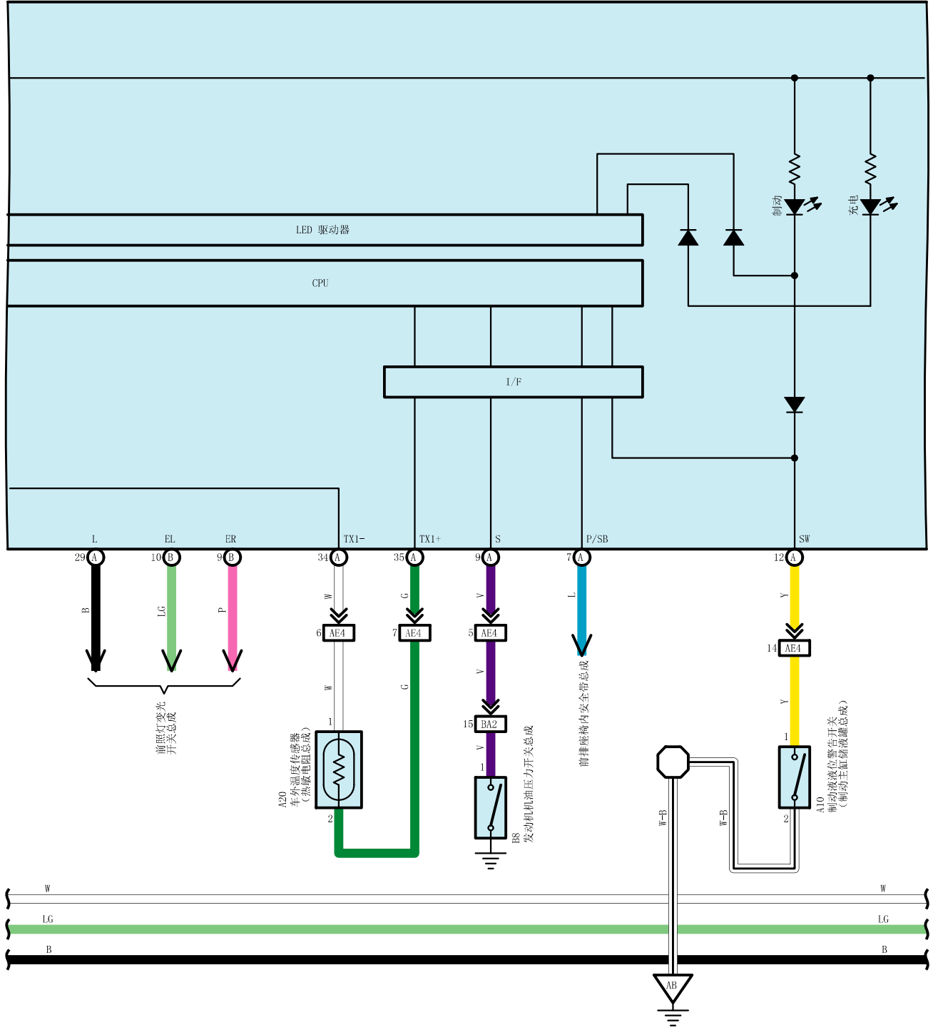
E55 (A), E59 (B) 组合仪表总成
